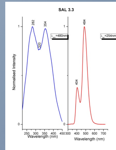
Spectre PLE si PL ale SAL:Eu 2+
