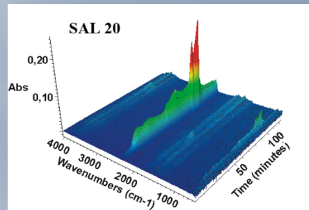
Spectrul FTIR al gazelor eliberate in analiza termica a precursorului
